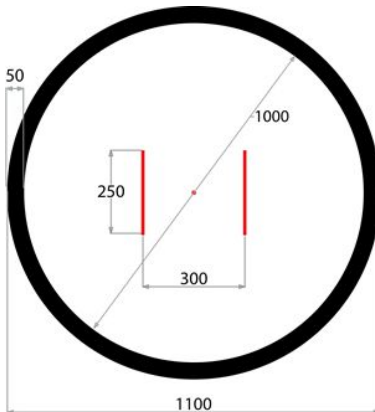
Рис. 2.1. Общий вид поля с размерами
